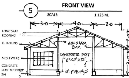
5 FRONT VIEW SCALE: 1:125 M.
