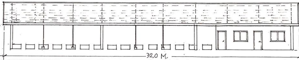
4 RIGHT SIDE VIEW SCALE: 1:125 M.
